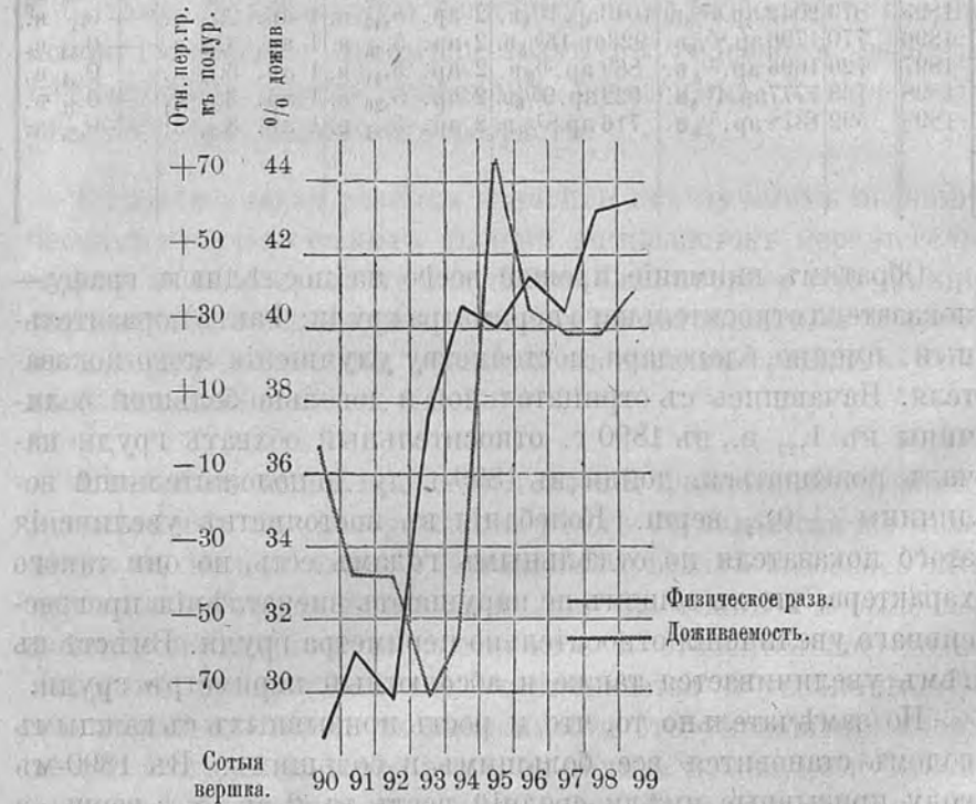
Диаграмма № 7-й. Физическое развитіе съ 1890 по 1899 г. и доживаемость до призывного возраста.
