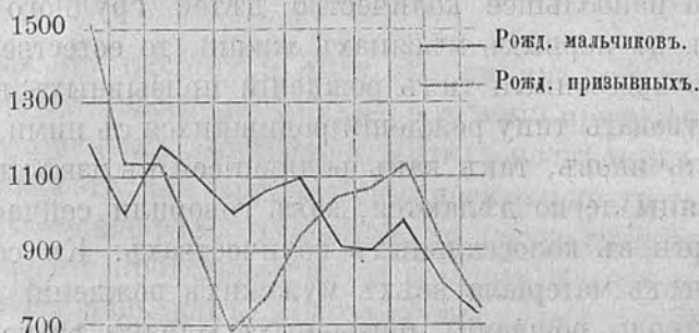
Діаграмма № 3. Соотнош. рожд. мальчиковъ и рожденій призывныхъ.
