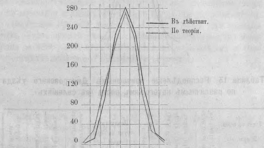
Діаграмма № 5-й. Законъ бинomialности роста призывныхъ.
