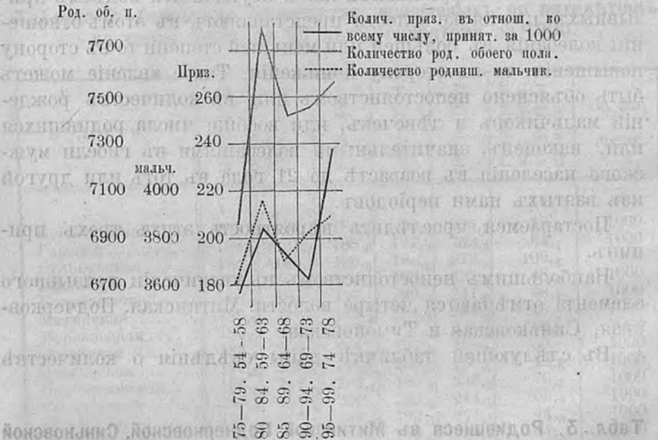
Діаграмма № 1. Число призывныхъ и родившихся.
