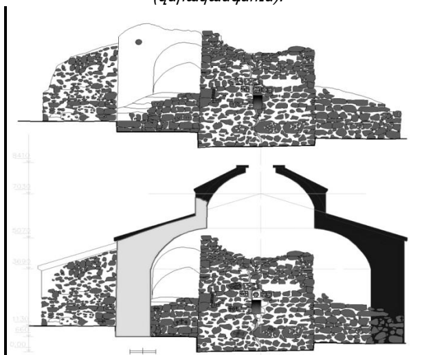
Գծ. 2. Գավիթ ժամատան ծածկի վերականգնումը:
