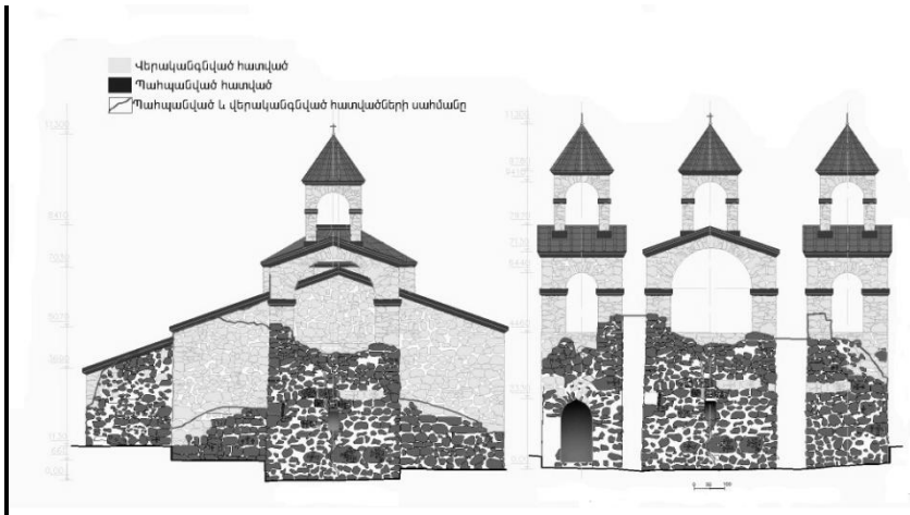
Պճ. 3. Զանգակատան արևմտյան ճակատի վերականգնումը:
