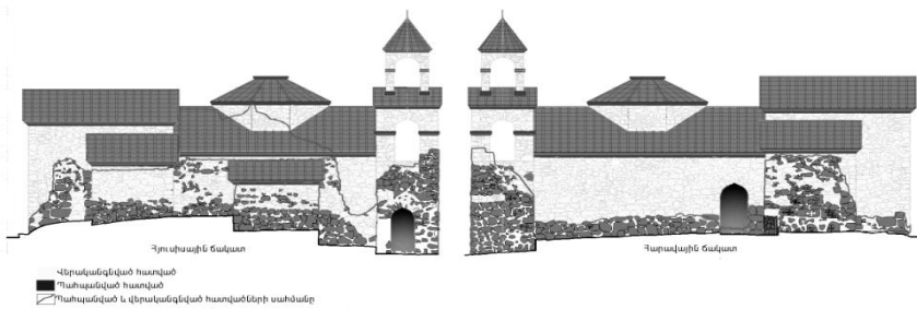
Գծ. 1. Շինությունների հիմնական խմբի հյուսիսային և հարավայն ճակատները (վերականգնում):
