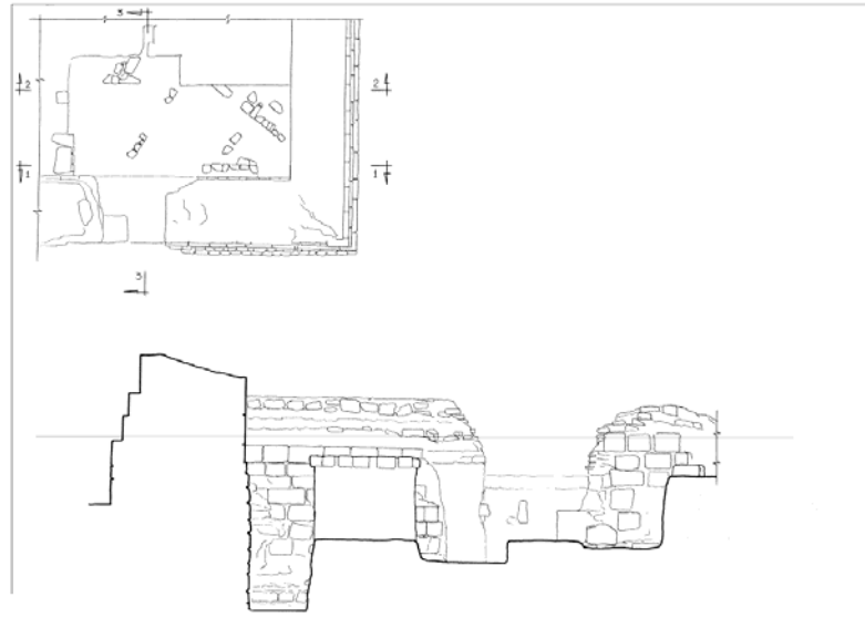
Դվինի Մայր տաճարի հարավային պատի արևմտյան հատվածի ներքին տեսքը: Չափագրությունը՝ Արմեն Հակոբյանի
