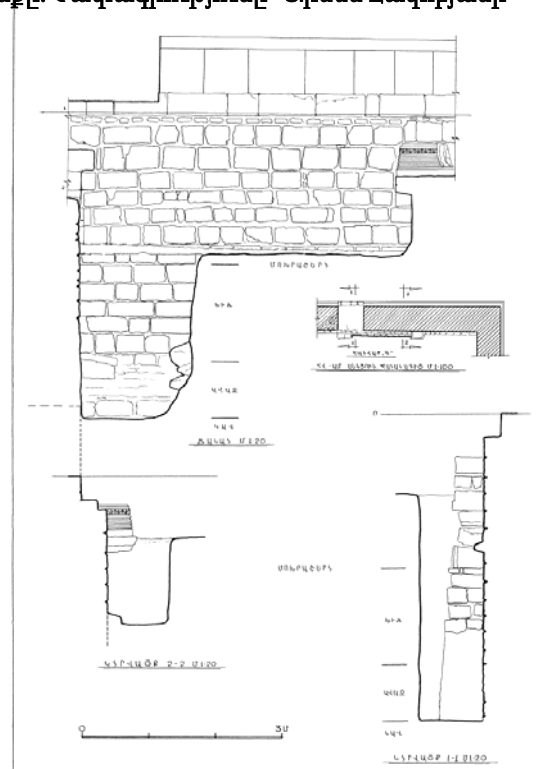
Դվինի Մայր տաճարի հարավային պատի արևմտյան հատվածի ներքին տեսքը: Չափագրությունը՝ Արմեն Հակոբյանի
