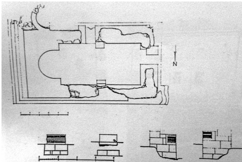
Եկեղեցու հատակագիծը (ճարտարապետ Ա. Տեր-Մինասյան)
