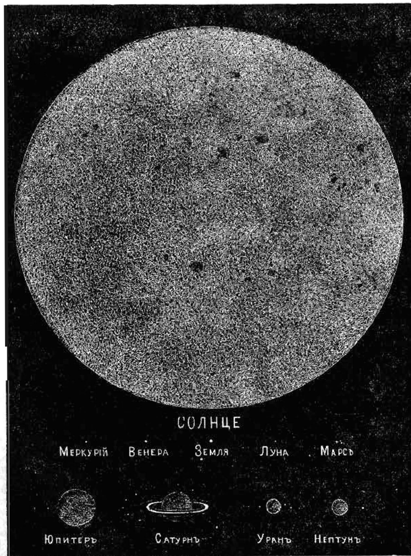
Сравнительная величина Солнца и планет солнечной системы.
