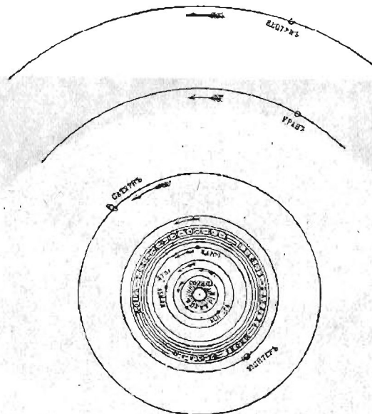
СОЛНЕЧНАЯ СИСТЕМА
