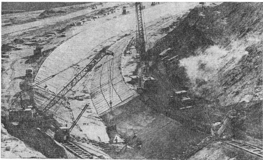
Досрочно завершено строительство 3-й очереди Большого Ставропольского канала, 1979 г.
