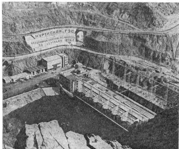
Нуркенская ГЭС. 30 сентября введена на полную мощность — 2700 тыс. киловатт.
