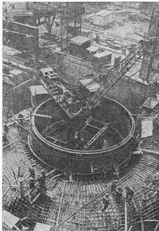
Сооружение спиральной камеры 3-го гидроагрегата Саяно-Шушенской ГЭС.
