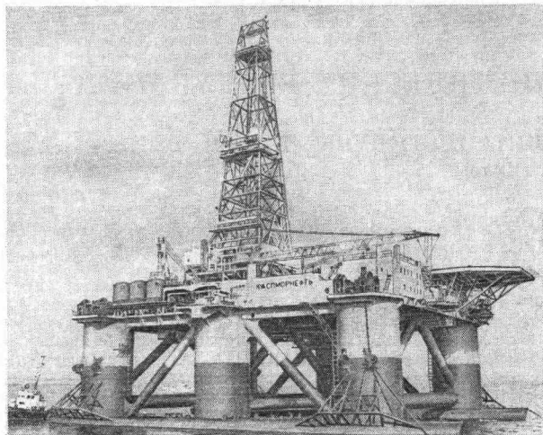
Полупогруженная установка «Каспморнефть» пополнила в 1979 г. флотилию плавучих буровых, ведущих поиски нефти в Каспийском море. Она способна вести бурение на участках глубиной 200 м (второе больше, чем доступно обычным буровым).
