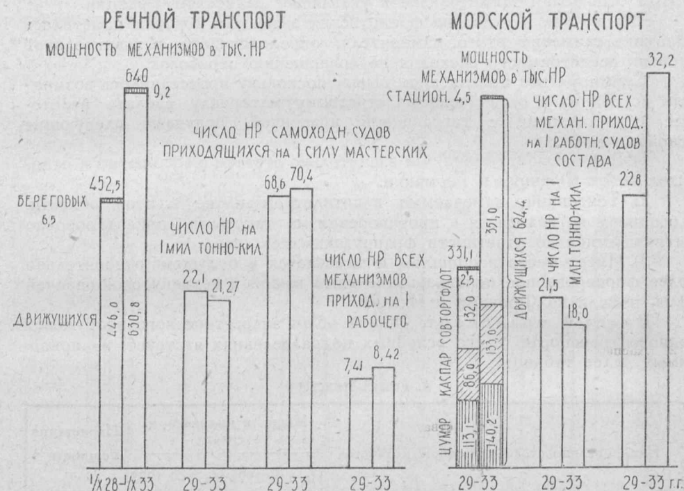
Динамика энерговооружения водного транспорта за пятилетие 1928/29—1932/33.
