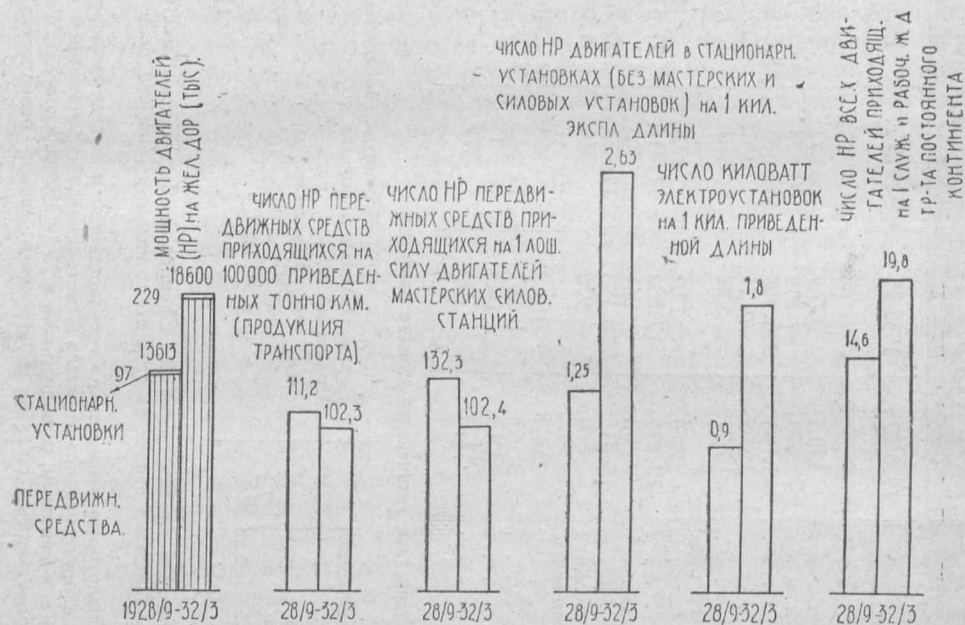
Динамика Энерговооружения ж.-д. транспорта за пятилетие 1928/29—1932/33.
