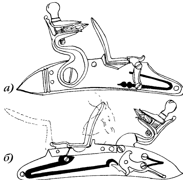
Кремнево-ударный замок: а) лицевая сторона; б) оборотная сторона.
