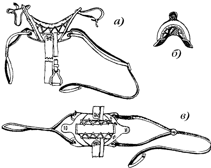
Строевое седло легкой кавалерии в первой половине XIX века: а) ленчик с подпругами, путищами, пахвями и паперстями, троками на передней и задней луке (вид сбоку); б) ленчик без ремней (вид сзади); в) ленчик с подпругами, путищами, пахвями и паперстями (вид сверху).
