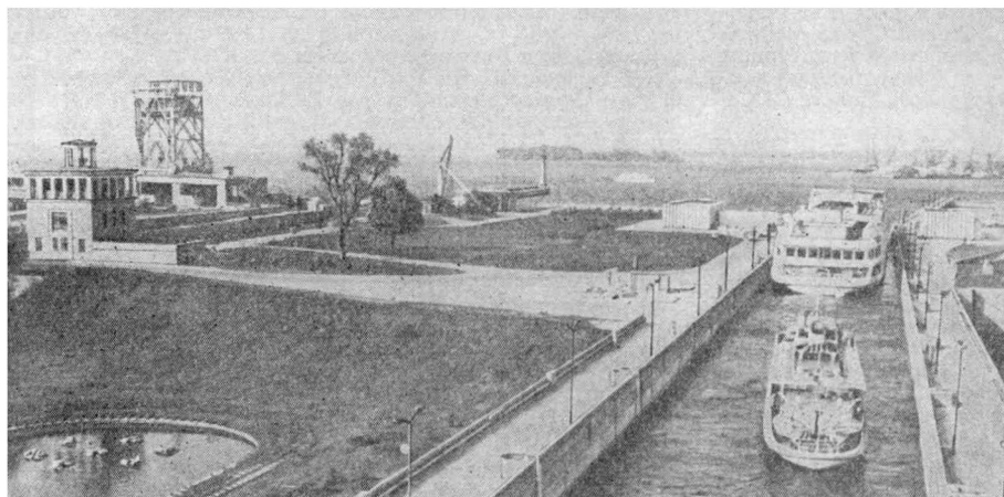
Новый однокамерный шлюз Днепровской ГЭС им. В. И. Ленина.
