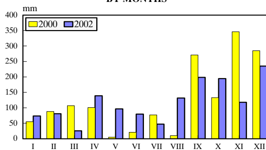
Граф. 2. 4. ВИСИНА ПАДАВИНА У ПОДГОРИЦИ ПО МЕСЕЦИМА PRECIPITATION IN PODGORICA BY MONTHS
