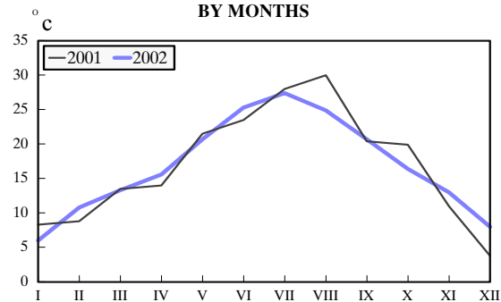
Граф. 2. 2. ТЕМПЕРАТУРА ВАЗДУХА У ПОДГОРИЦИ ПО МЕСЕЦИМА AIR TEMPERATURE IN PODGORICA BY MONTHS
