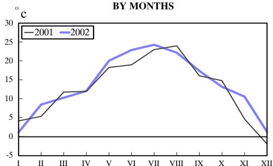
Граф. 2. 1. ТЕМПЕРАТУРА ВАЗДУХА У БЕОГРАДУ ПО МЕСЕЦИМА AIR TEMPERATURE IN BELGRADE BY MONTHS
