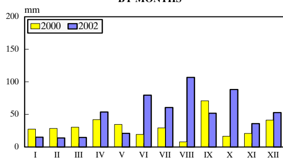
Граф. 2. 3. ВИСИНА ПАДАВИНА У БЕОГРАДУ ПО МЕСЕЦИМА PRECIPITATION IN BELGRADE BY MONTHS
