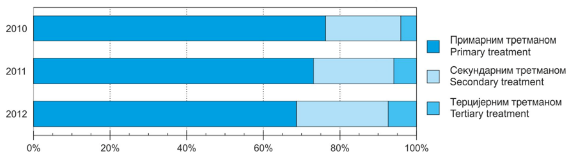
Граф. 11.4. УДЕО ОТПАДНИХ ВОДА ПРЕМА ВРСТИ ТРЕТМАНА, 2010-2012. SHARE OF WASTEWATER BY TREATMENTS, 2010-2012
