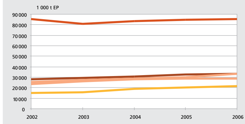
Gráfico 4.3.2 - Evolução da oferta interna de energia - Brasil - 2002-2006
