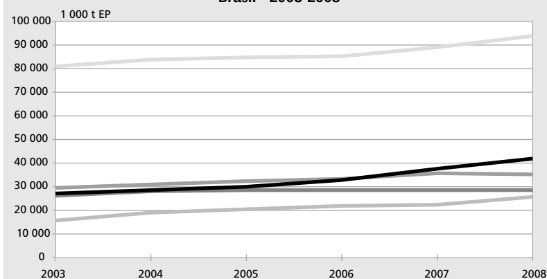
Gráfico 4.3.2 - Evolução da oferta interna de energia Brasil - 2003-2008
