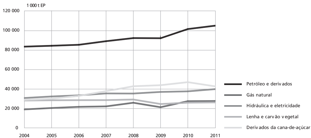
Gráfico 4.3.2 Evolução da oferta interna de energia - Brasil - 2004-2011
