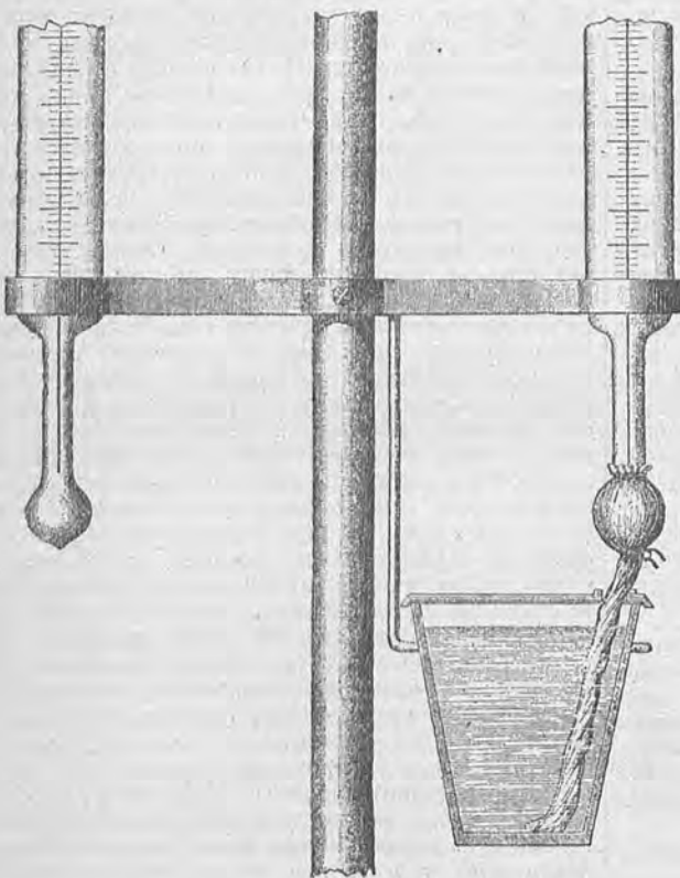
Психрометръ.
