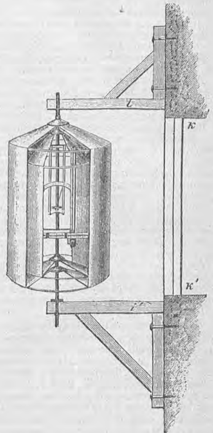
Клѣтка для помѣщенія метеорологическихъ приборовъ.
