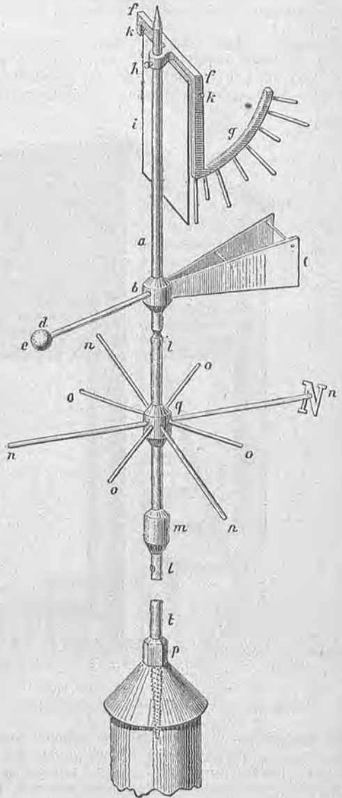
Флюгеръ.
