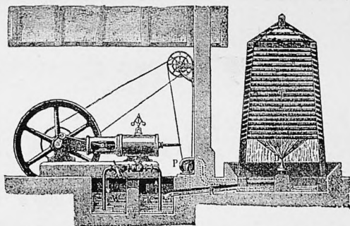
Устройство конденсаціи охлажденія воды въ башнѣ.
