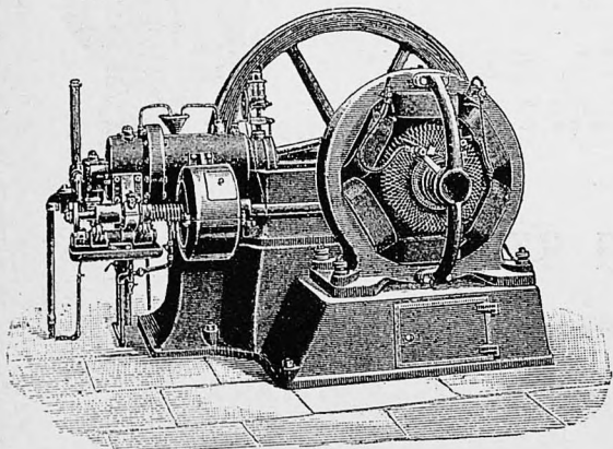
Газодвижущаяся динамо Кертинга.
