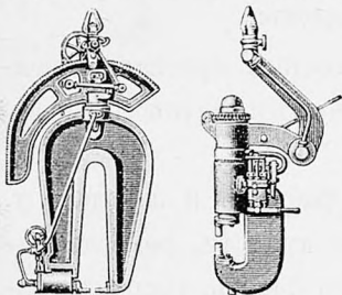
Ножницы для обрѣзыванія металлическихъ листовъ.
