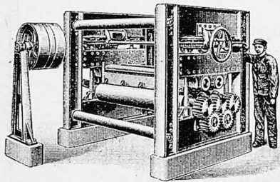
Машины для выправки листовъ желѣза до 40 mm.
