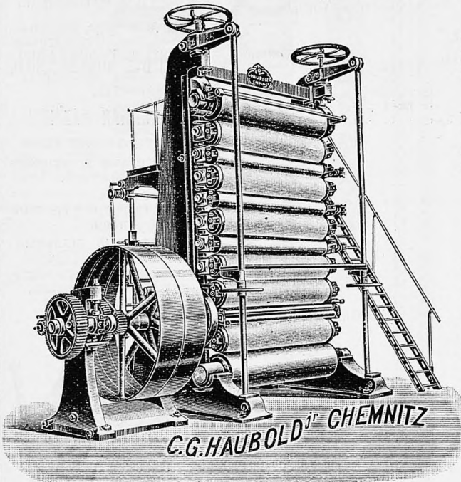
Каландръ съ 12 вилками.
