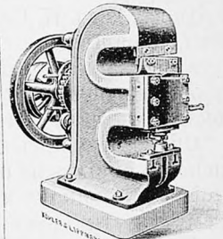
Машины для выправки листового желѣза до 40 mm.
