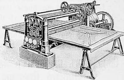
Машины для выправки листового желѣза до 40 mm.
