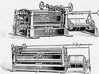
Строгательныя машины для обдѣлки кромокъ листового желѣза.
