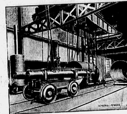
Комб. пробойныя машины для и ножицы желѣзныхъ наугольниковъ.
