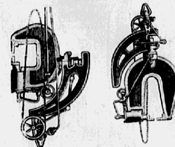
Комб. прокатывающія маши- ны и ножицы.
