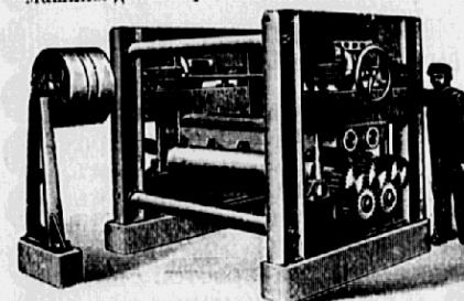
Машины для выправки листового желѣза до 40 мм.
