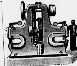
Комб. пробойныя машины для и ножицы желѣзныхъ наугольниковъ.
