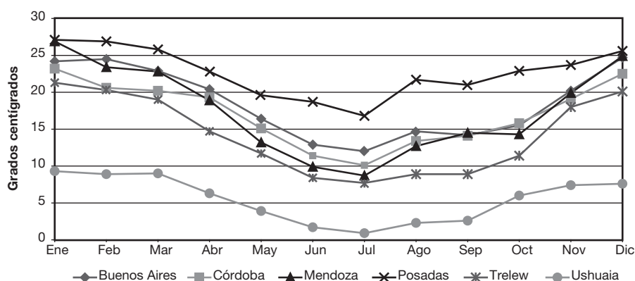
Gráfico 2. Temperaturas medias mensuales por estación meteorológica. Año 2015
