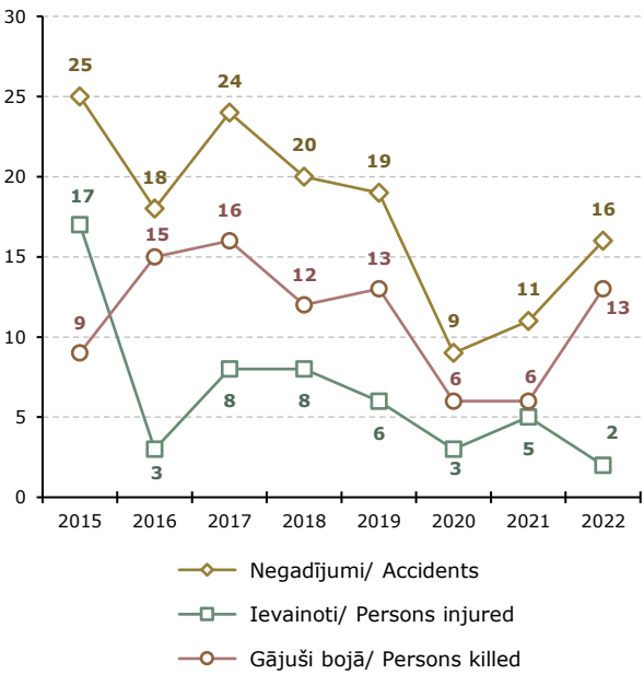
Nopietnu dzelzceļa negadījumu skaits Number of rail accidents
