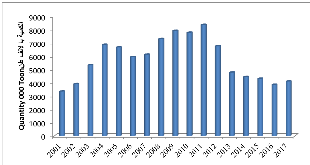
شكل 1.2.11 كمية بضائع الترانزيت المارة بالأراضي الأردنية، 2001-2017 (بالألف طن) Figure 11.2.1 Quantity of Transit Commodities Passing Through Jordan, 2001 –2017 (000Ton)
