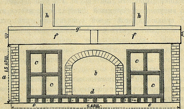
Рис. 3-й. Сушилка Ошанина.
