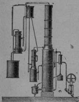
Привилегированный брагоперегонный ректификационный аппаратъ.
