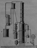
Привилегированный брагоперегонный ректификаціонный аппаратъ.
