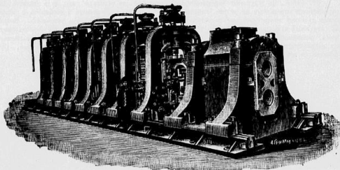
Машина и Бадонный станъ „Дуо“ 850 м/м фут. изготовленныя Екатеринославскимъ Машиностроительнымъ заводомъ на (Амуръ).
