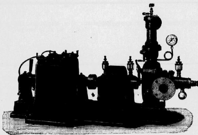
Паровая турбо-динамо, завода Де-Лавали въ Стокгольмѣ. Представитель В. Девенсонъ, Екаторинославѣ.
