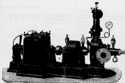
Паровая турбо-динамо, завода Де-Лавала въ Стокгольмъ. Представитель В. Левенеонъ, Екатеринославъ.
