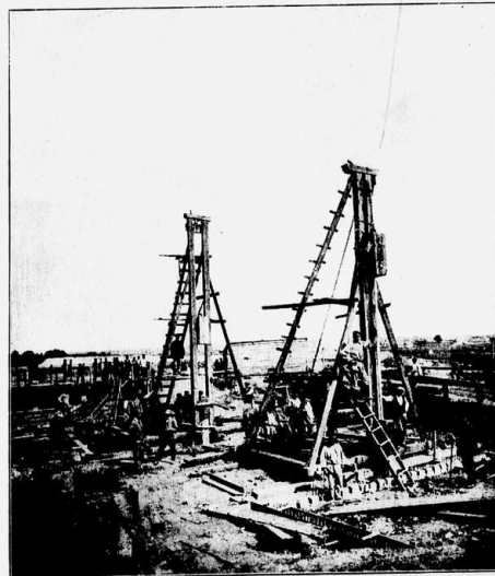
Забивка желѣзобетонныхъ свай по системѣ Геннебикъ при постройкѣ моста въ Тритузныхъ хуторахъ Екатеринославской губерніи и уѣзда; строители инженеры Моникуръ и Эггеръ въ Екатеринославѣ.
