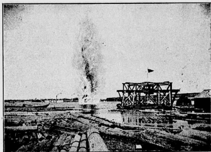
Взрывъ камня во время работъ по очисткѣ фарватера на рѣкѣ Днѣпрѣ, близъ г. Енатеринослава.
