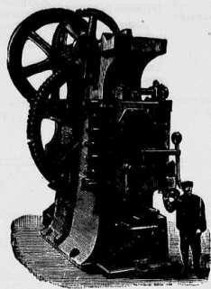
Изготовленный заводомъ, Краматорскаго Металлургическаго О-ва въ Краматорской, Харьковской губ.
