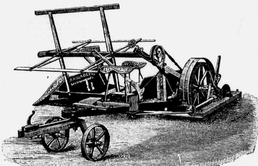
УГЛЕПОДЪЕМНАЯ МАШИНА И ЖАТКА, изготовленные машиностроительнымъ и чугунолитейнымъ заводомъ Бр. ЛАЩАВЕРЪ въ Екатеринбургѣ.
