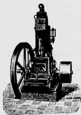
Керосиновые двигатели (вертикальный и горизонтальный) завода ОТТО-ДЕЙЦЪ.
