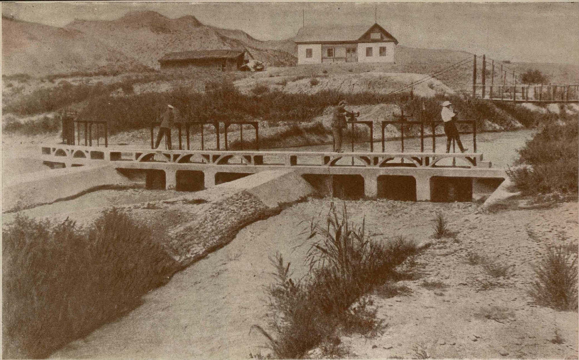
Водные сооружения на реке Турьян-чай, Агдашского района
