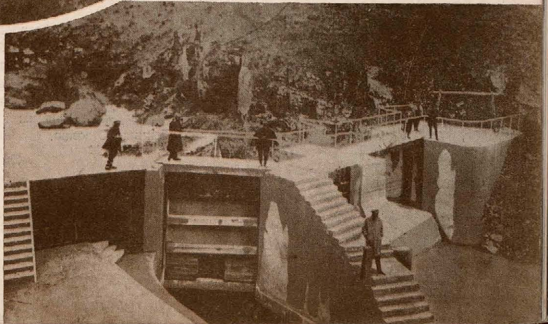
Шлюзы Нухинской гидро-электростанции.
