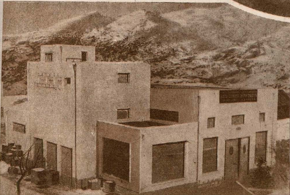
Зурнабадская гидро-электростанция.
