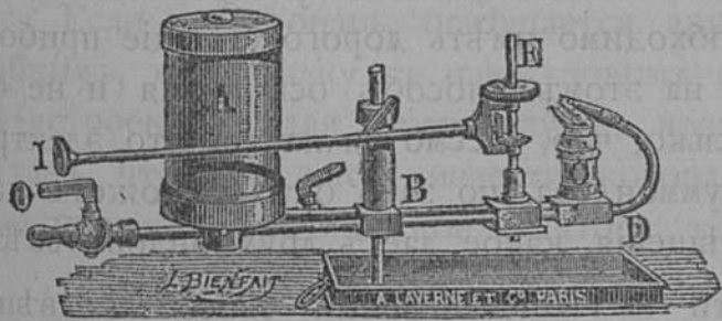
Рис. 36. Горѣлка спирто-кислородная.
