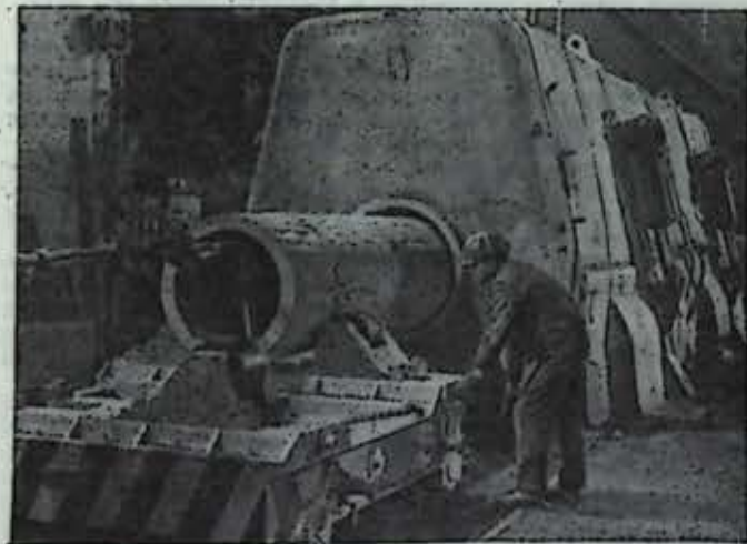
Рис. 1. Центробежная машина для отливки заготовок диаметром 0,6—1,5 м и длиной до 9 м из стали, чугуна и бронзы.
