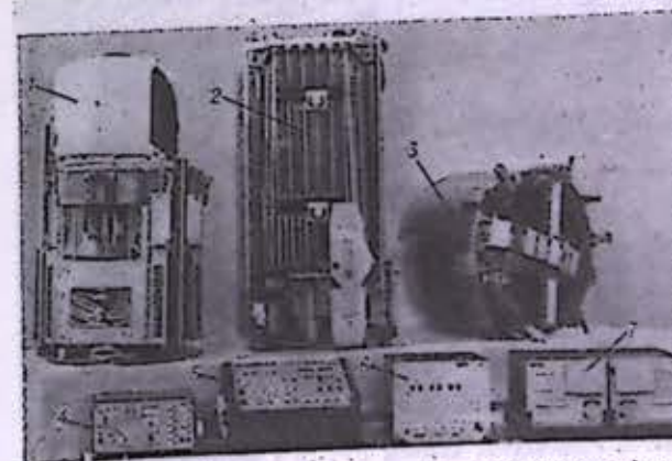
Рис. 2. Аппаратура КРТ-10 в транспортном (сложенном) состоянии: 1 — фокальный контейнер с опорами; 2 — зеркало антенны; 3 — механизм крепления антенны к станции; 4 — антенны; 5 — пульт управления; 6 — блок времени; 7 — низкочастотные блоки радиометров.
