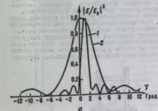
Рис. 7. Диаграммы направленности антенны KPT-10 в вертикальной (а) и горизонтальной (б) плоскостях в диапазоне длин волн 12 см (кривые 1) и 72 см (кривые 2): |E/E_0|^2 — относительная мощность принятого сигнала; \gamma и \beta углы, отсчитываемые от продольной оси станции «Салют-6» соответственно в вертикальной и горизонтальной плоскостях.
