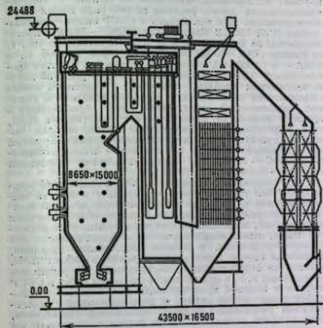
Схема парогенератора ТП-101.
