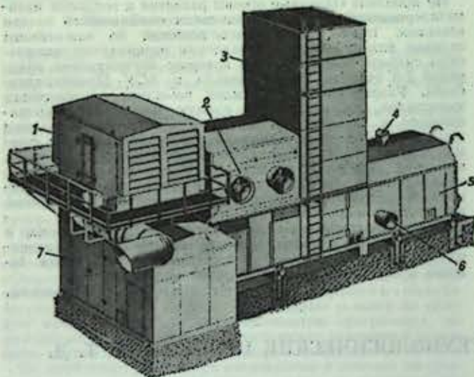
Газоперекачивающий агрегат ГПА-Ц-6,3: 1 — воздухоочистительное устройство; 2 — блок маслоохладителей; 3 — выхлопная шахта; 4 — дефлектор; 5 — блок турбоагрегата; 6 — пускательный патрубок; 7 — всасывающая камера с контейнером автоматики.
