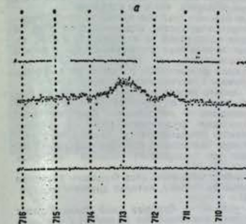
Рис. 6. Примеры записей телеметрической информации, переданной на Землю в процессе измерения характеристик антенны KPT-10: а — запись сигнала от дискретного источника радионизлучения Кассиопея-А в 12-сантиметровом диапазоне волн; б — запись сигнала от Солнца в 72-сантиметровом диапазоне волн.
