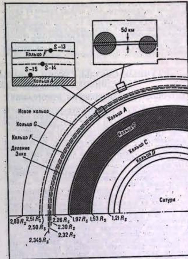
Рис. 20. Положение спутников S-10, S-11, S-13 (на рис. в верхнем правом квадрате S-10 — слева, S-11 — справа), S-14 и S-15 относительно колец Сатурна.
