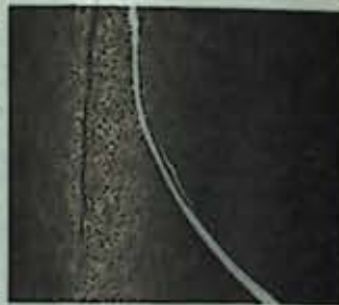
Рис. 9. Переплетение «прядей» в кольце F (снимок с расстояния 750 тыс. км).
