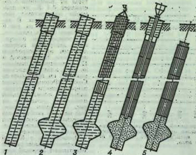
Рис. 1. Схема технологического цикла сооружения наклонных буровых свай с уширенным основанием при глубине воды до 8–10 м: 1 — бурение ствола скважины под защитой глинистого раствора; 2 — разбуривание уширения в основании скважины; 3 — опускание арматурного каркаса; 4 — заполнение скважины подводным бетоном; 5 — готовая свая.
