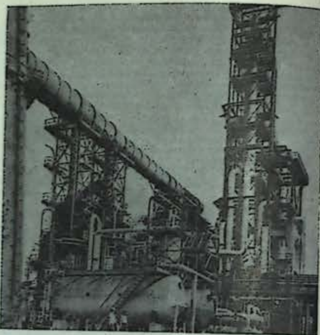
Установка каталитического риформинга на Новобаккинском нефтеперерабатывающем заводе им. Владимира Ильича.
