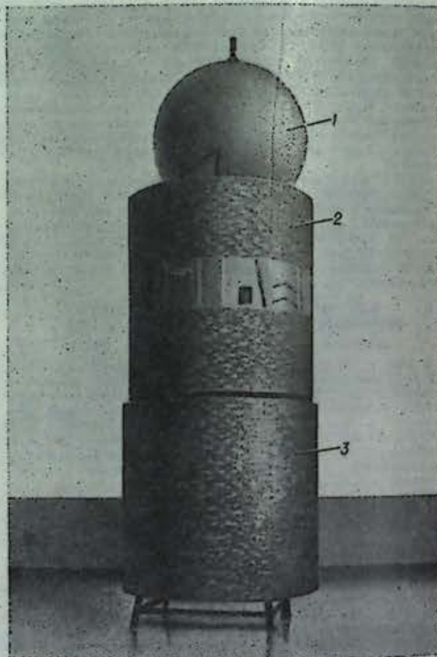
Рис. 2. ИСЗ SBS-1: 1 — ретрансляционная антенна (в рабочем положении); 2 — корпус ИСЗ с установленными на нем солнечными батареями; 3 — цилиндр с солнечными батареями (сдвинут в рабочее положение).
