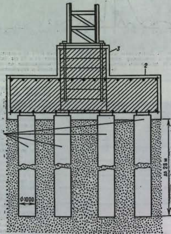
Рис. 2. Конструкция фундамента на буронабивных сваях диаметром 600–1200 мм: 1 — свая; 2 — ростверк; 3 — несущая колонна.
