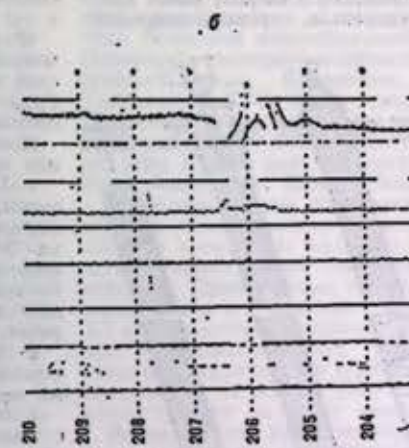
Рис. 6. Примеры записей телеметрической информации, переданной на Землю в процессе измерения характеристик антенны KPT-10: а — запись сигнала от дискретного источника радионизлучения Кассиопея-А в 12-сантиметровом диапазоне волн; б — запись сигнала от Солнца в 72-сантиметровом диапазоне волн.
