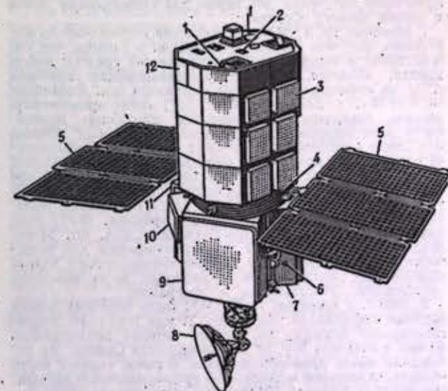
Рис. 1. ИСЗ SMM: 1 — солнечные датчики грубой ориентации; 2 — солнечный датчик точной ориентации; 3 — жалюзи системы терморегулирования; 4 — переходник; 5 — панели солнечных батарей; 6 — выступ для захвата спутника дистанционным манипулятором МТКК «Спейс шаттл»; 7 — блок оборудования системы ориентации; 8 — антенна (вес 11,3 кг, диаметр 1,27 м) для связи с Землей через спутник-ретранслятор TDRSS; 9 — блок оборудования связи и обработки информации; 10 — устройство управления и обработки сигналов; 11 — блок оборудования системы электропитания; 12 — блок полезной нагрузки.
