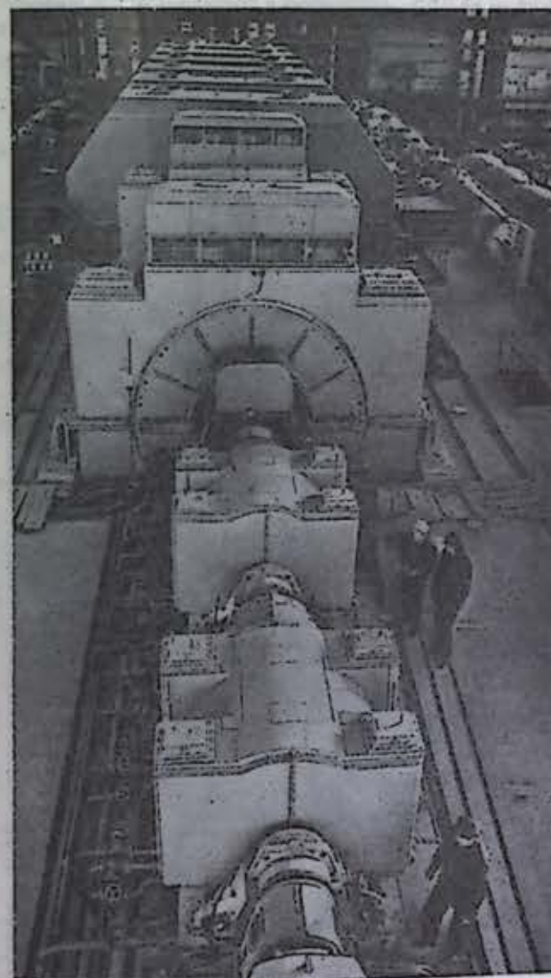
Костромская ГРЭС. Энергоблок мощностью 1 млн. 200 тыс. кВт.
