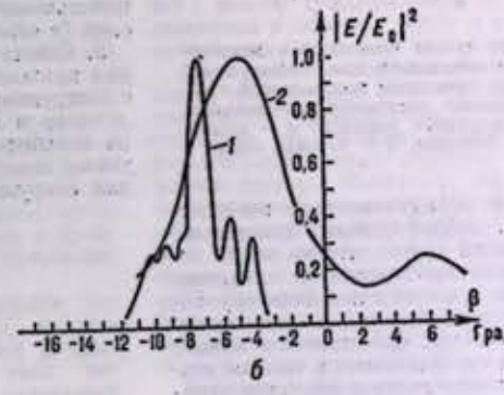
Рис. 7. Диаграммы направленности антенны KPT-10 в вертикальной (а) и горизонтальной (б) плоскостях в диапазоне длин волн 12 см (кривые 1) и 72 см (кривые 2): |E/E_0|^2 — относительная мощность принятого сигнала; \gamma и \beta углы, отсчитываемые от продольной оси станции «Салют-6» соответственно в вертикальной и горизонтальной плоскостях.
