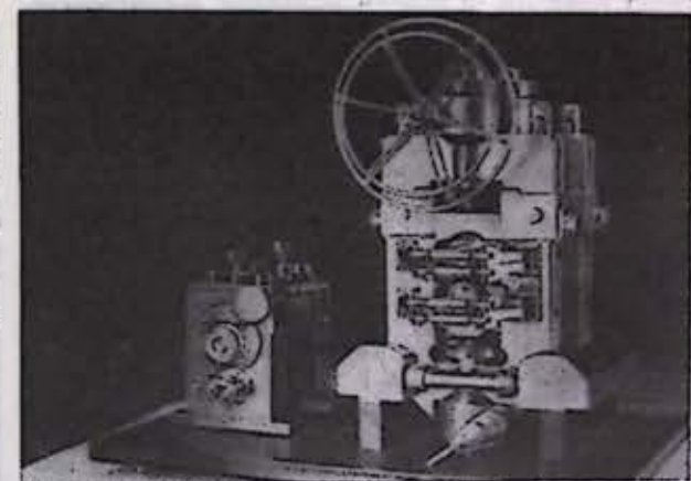
Рис. 2. Сравнение габаритов предварительно-напряженной (слева) и станниной рабочих клеток стана «250» (общий вид моделей, М 1:10).
